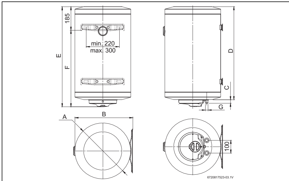
Fig. 2 Dimensions en mm (montage vertical)
