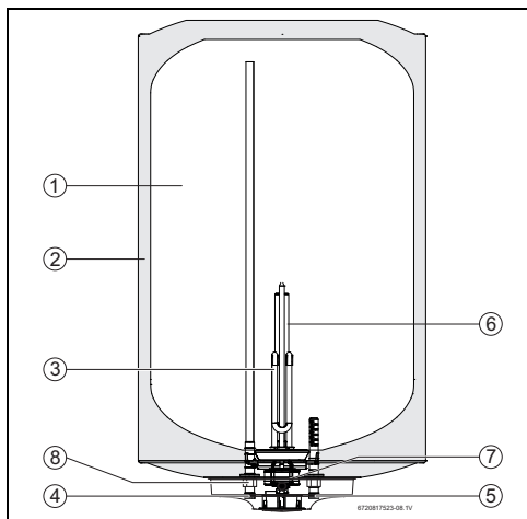
Fig. 4 Composition du ballon (exemple Elacell)
