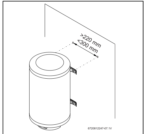
Fig. 7 Montage vertical
