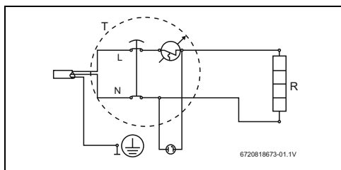
Fig. 5 Schéma de raccordement
