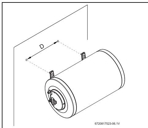
Fig. 8 Montage horizontal
