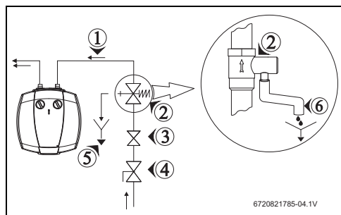
Fig. 10 Raccordement d'eau
