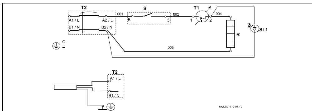
Fig. 5 Schéma de raccordement
