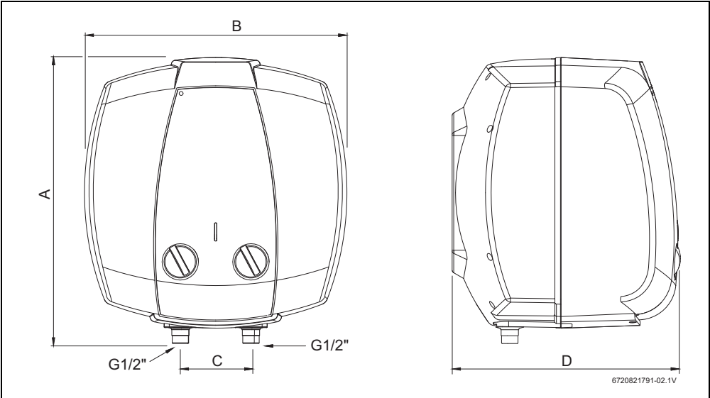
Fig. 2 Dimensions en mm
