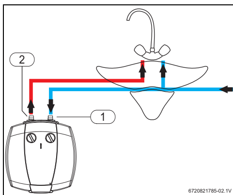
Fig. 8 Installation sous le lavabo
